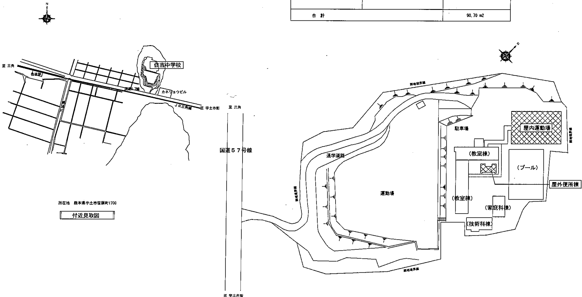
配置図 1/600
