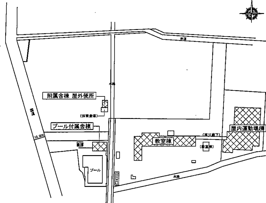
配置図 1/800
