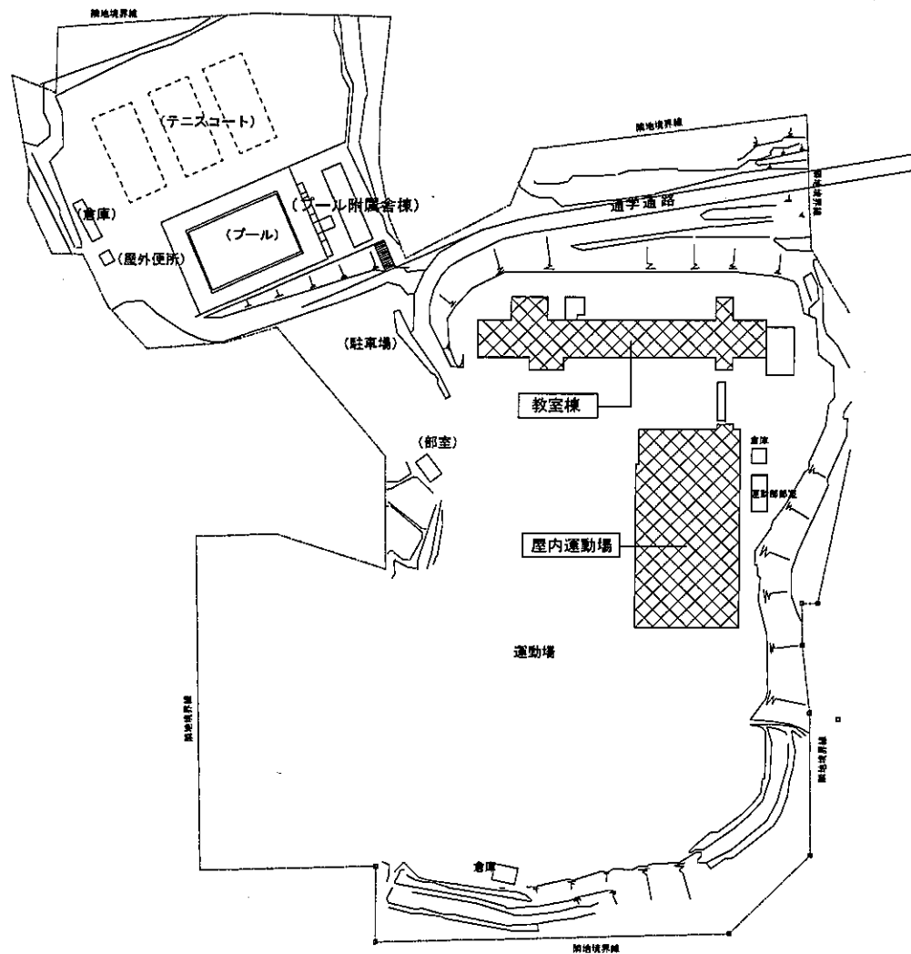
配置図 1/800
