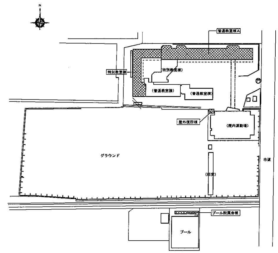
配置図 1/700
