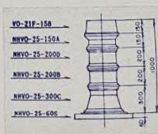
仕切弁ボックス詳細図
