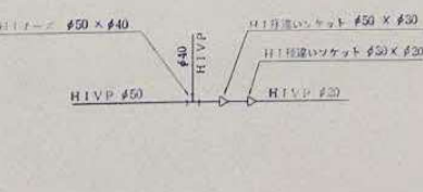
D 詳図
