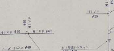
E 詳図
