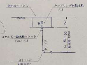
散水栓詳細図
