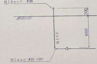
散水栓詳細図
