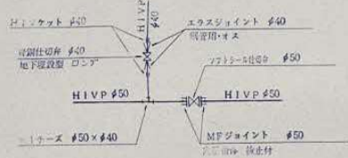
B 詳図
