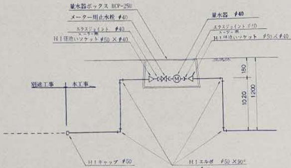
B 詳図
